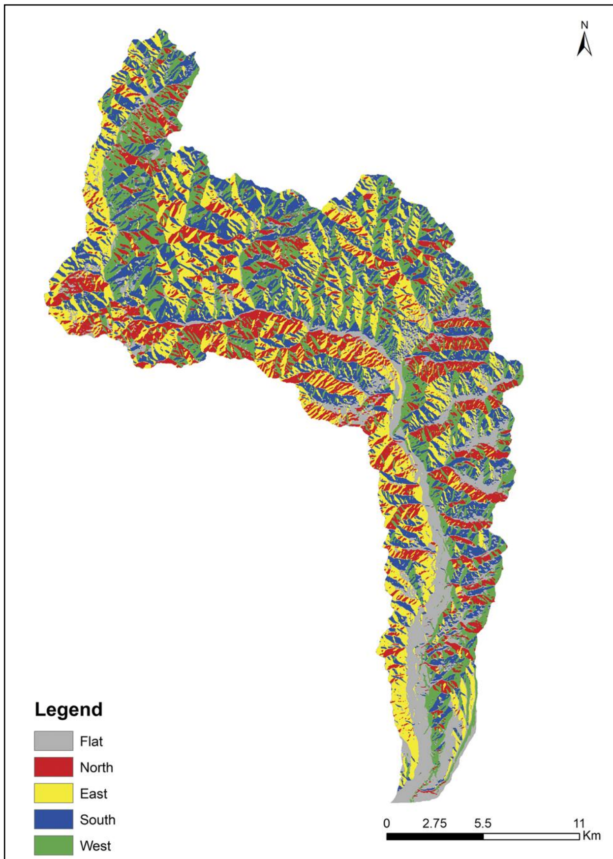
Fig. 20. The slope exposure map of Slănicul de Buzău Basin.
