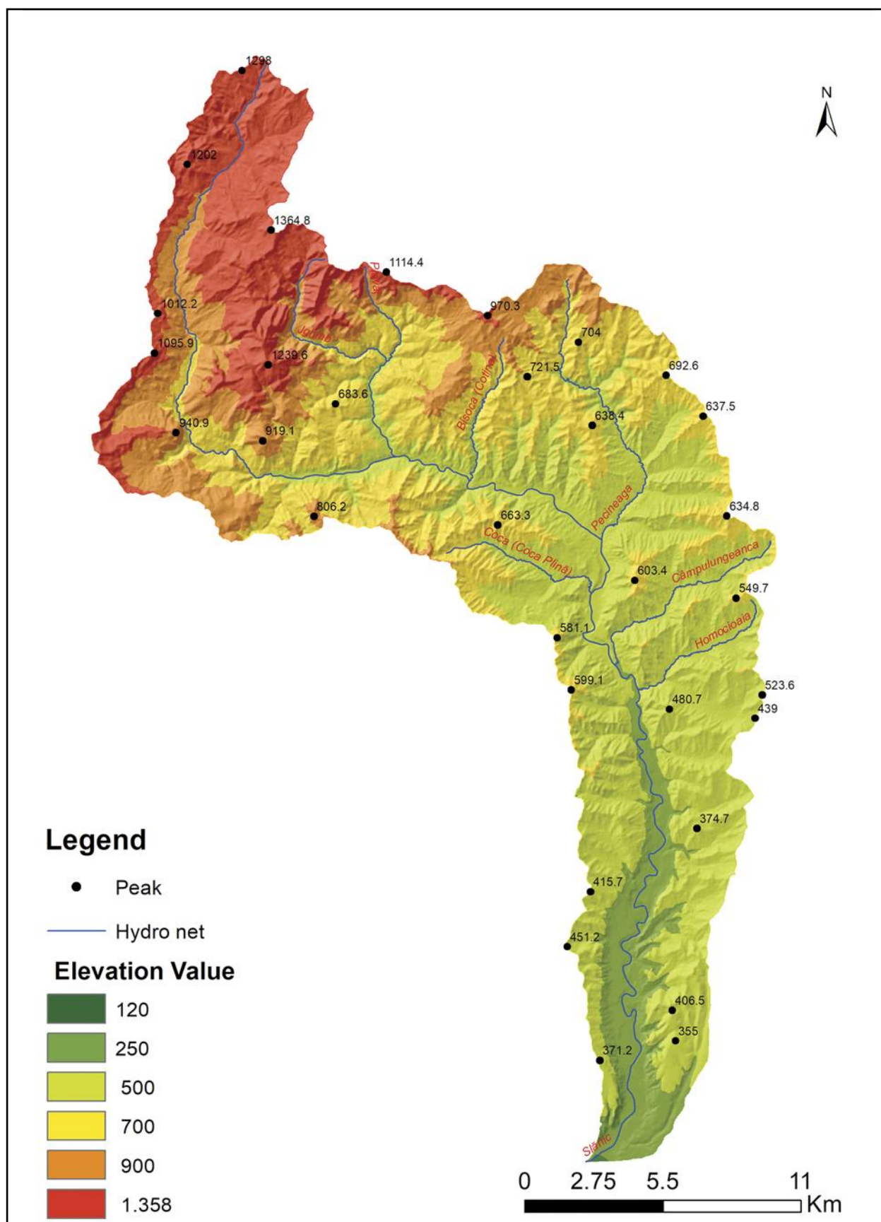
Fig. 21. Hypsometric map of the Slănicul de Buzău Basin.
