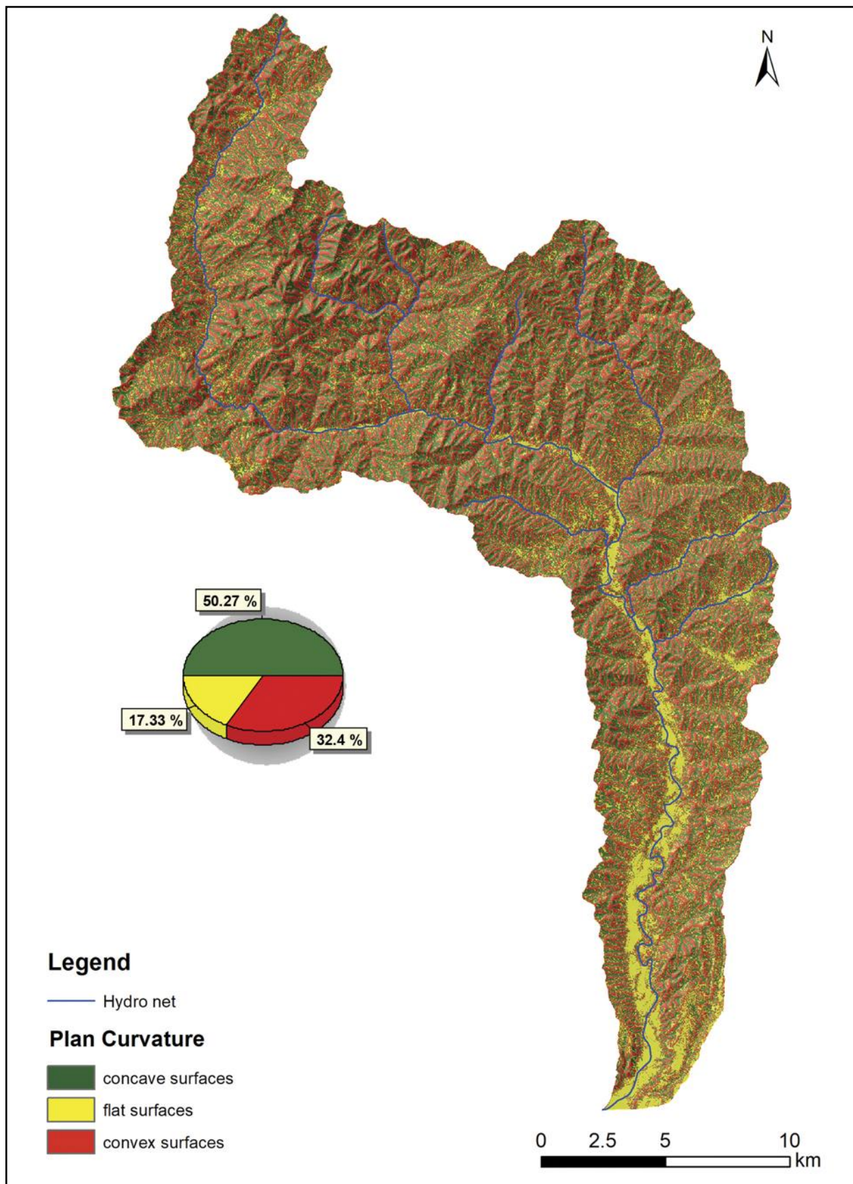
Fig. 22. Plan curvature map of the Slănicul de Buzău Basin.
